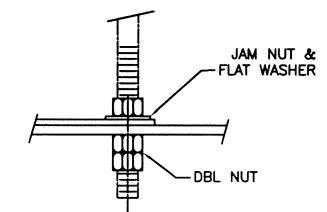
DETAIL 28-F SCALE: 1 1/2" = 1'-0"
